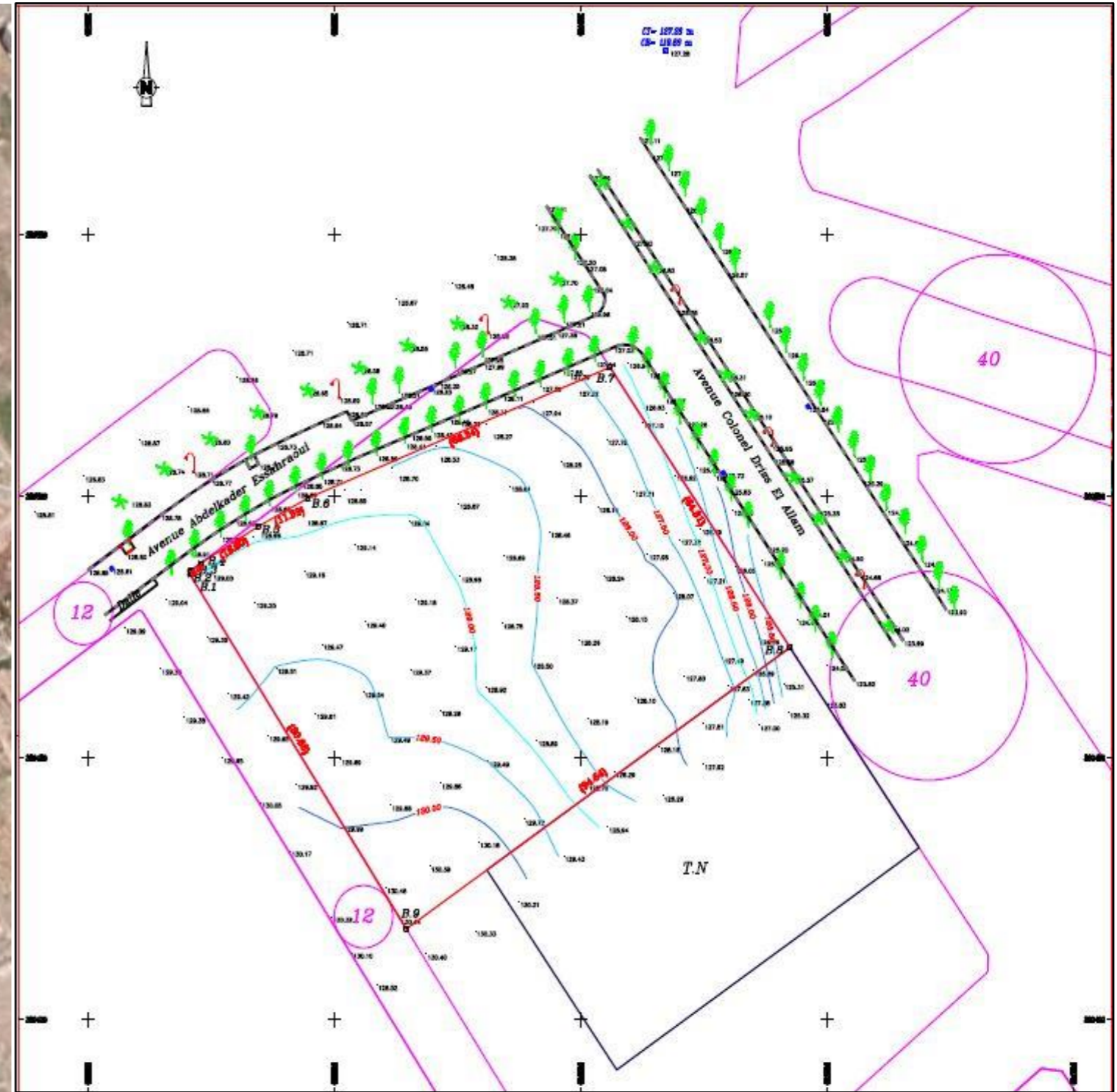
EXTRAIT DU PLAN COTE
